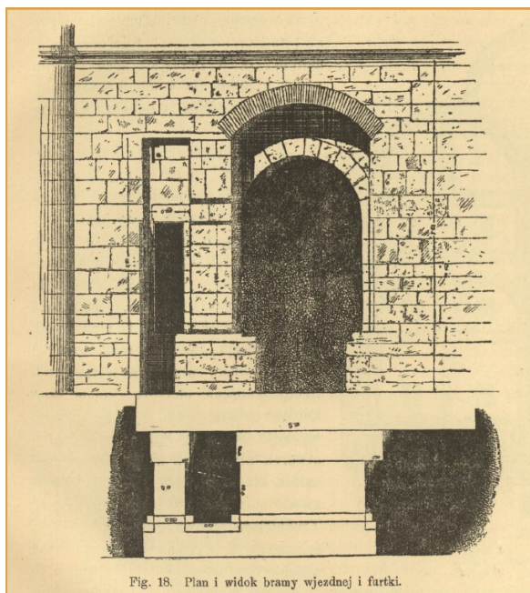
Fig. 18. Plan i widok bramy wjazdnej i furtki.
