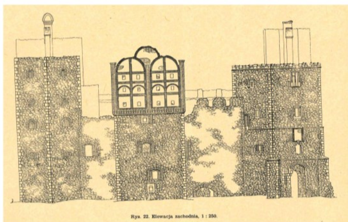
Rys. 22. Kłowacja zachodnia, 1 : 250.
