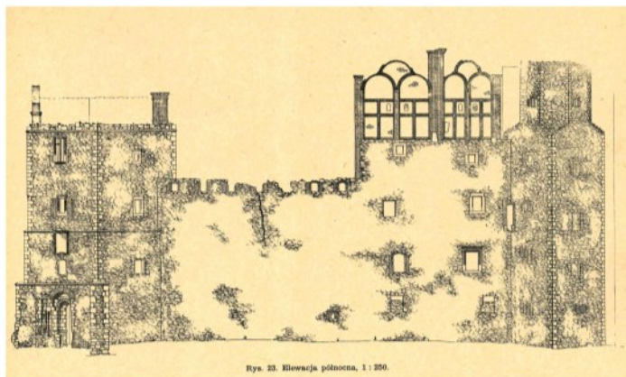
Rys. 23. Kłowacja północna, 1 : 250.
