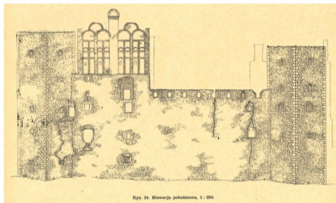
Rys. 24. Kłowacja południowa, 1 : 250.
